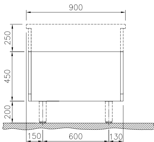
Boven aanzicht
